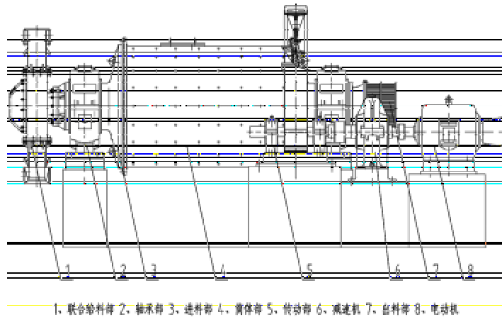
1. 联合给料部 2. 轴承部 3. 进料部 4. 筒体部 5. 传动部 6. 减速机 7. 出料部 8. 电动机
